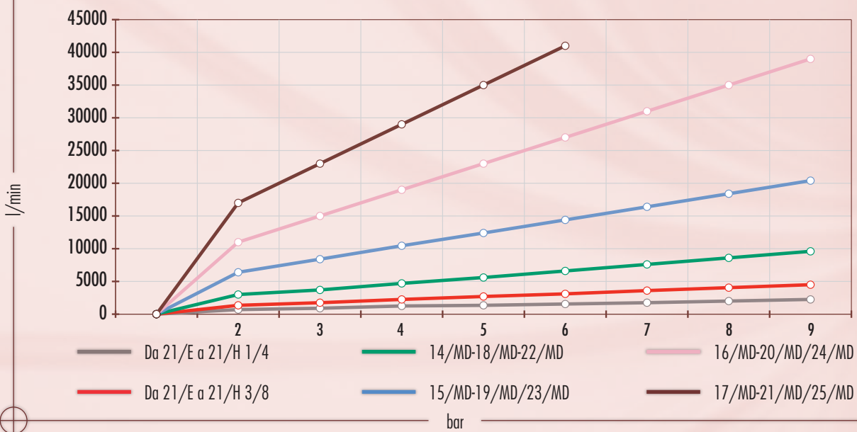
GRAFICO CONSUMO ARIA • AIR CONSUMPTION GRAPH GRAPHIQUE CONSOMMATION D'AIR
