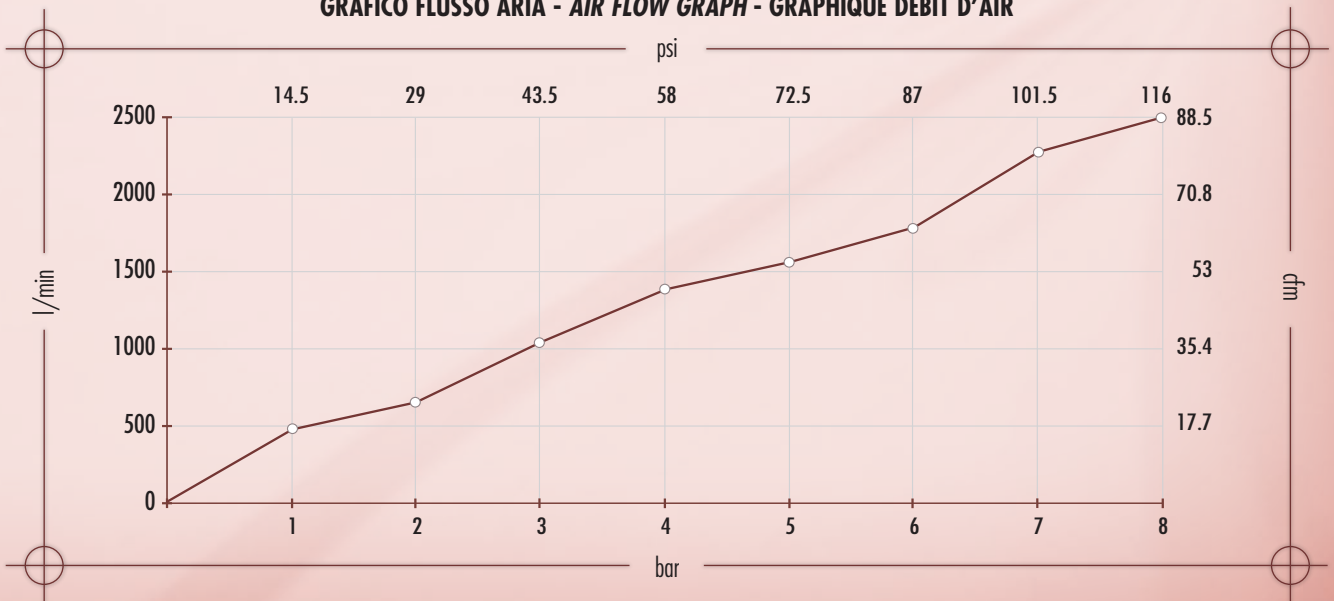
GRAFICO FLUSSO ARIA - AIR FLOW GRAPH - GRAPHIQUE DEBIT D'AIR
