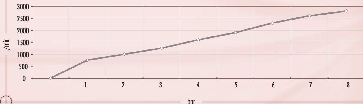
GRAFICO CONSUMO ARIA • AIR CONSUMPTION GRAPH GRAPHIQUE CONSOMMATION D'AIR
