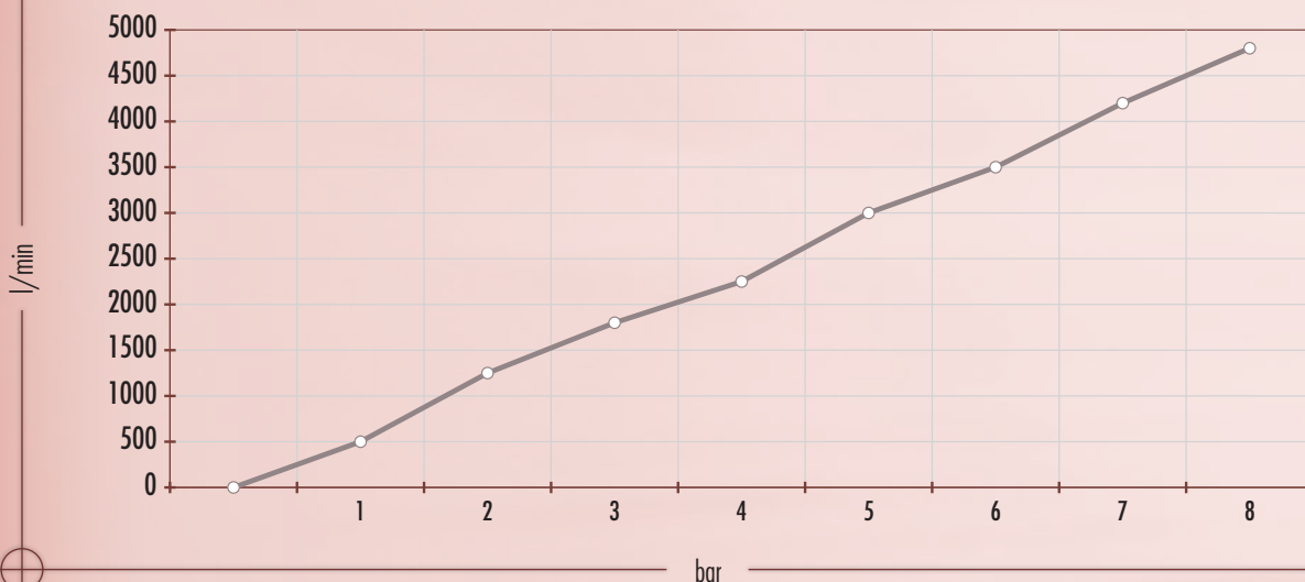
GRAFICO CONSUMO ARIA • AIR CONSUMPTION GRAPH GRAPHIQUE CONSOMMATION D'AIR
