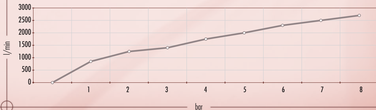
GRAFICO CONSUMO ARIA RUBINETTI A SFERE PER INNESTO A PROFILO GIAPPONESE • JAPANESE PROFILE BEARING TYPE QUICK COUPLER GRAPH GRAPHIQUE CONSOMMATION AIR RACCORDS A BILLES POUR EMBOUT JAPONAIS
