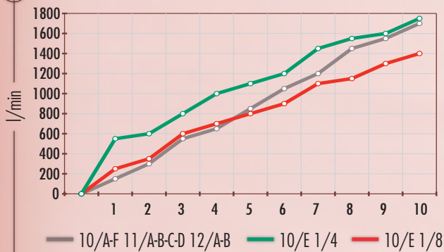
GRAFICO CONSUMO ARIA • AIR CONSUMPTION GRAPH GRAPHIQUE CONSOMMATION D'AIR
