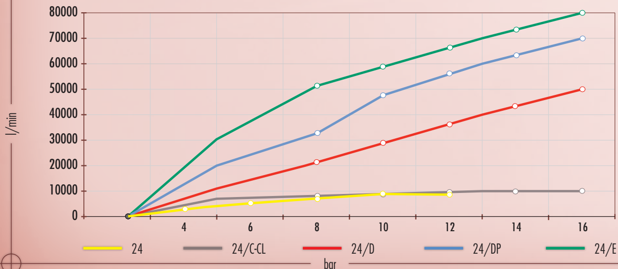
VALVOLE DI RITENUTA GRAFICO CONSUMO ARIA • NON RETURN VALVES AIR CONSUMPTION GRAPH GRAPHIQUE CONSOMMATION D'AIR CLAPET DE RETENUE
