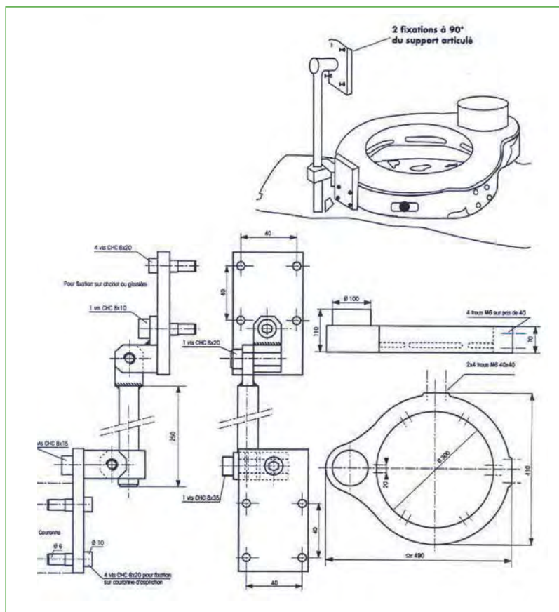
Corona aspirante Ø 300 mm
