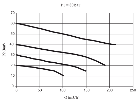
Curve di portata riferite all'ossigeno. Per l'azoto, i valori vanno moltiplicati per 1,07.
