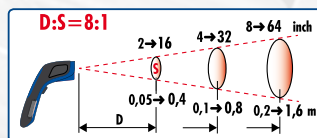
RISOLUZIONE OTTICA 8:1
